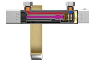
Термостатический картридж
