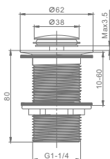
Артикул : R600.04.06 Донный клапан для раковины • Цвет - черный
