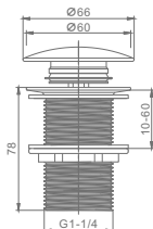
Артикул : R600.02 Донный клапан для раковины • Цвет - хром
