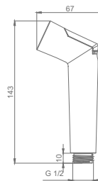
Артикул: R460.04.06 Гигиеническая лейка • Цвет - черный
