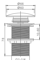
Артикул : R600.02.06 Донный клапан для раковины • Цвет - черный
