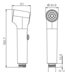
Артикул: R460.05.09 Гигиеническая лейка с клавишей регулировки воды • Цвет - графит
