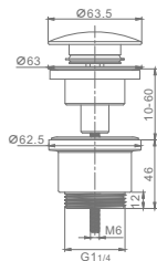
Артикул : R600.01.08 Донный клапан для раковины • Цвет - белый
