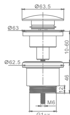
Артикул : R600.01 Донный клапан для раковины • Цвет - хром
