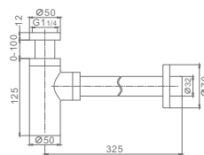
Артикул : R600.20.05 Сифон для раковины • Цвет - сатин
