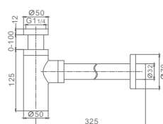
Артикул : R600.20 Сифон для раковины • Цвет - хром
