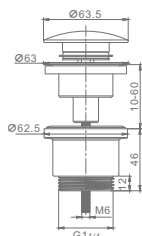
Артикул : R600.01.09 Донный клапан для раковины • Цвет - графит
