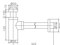
Артикул : R600.20.06 Сифон для раковины • Цвет - черный
