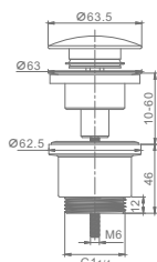
Артикул : R600.01.23 Донный клапан для раковины • Цвет - золото
