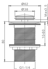
Артикул : R600.04 Донный клапан для раковины • Цвет - хром
