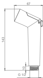
Артикул: R460.01 Гигиеническая лейка с клавишей регулировки воды • Цвет - хром
