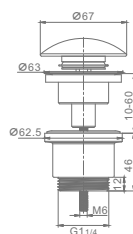
Артикул : R600.01.38 Донный клапан для раковины • Цвет - с керамической крышкой
