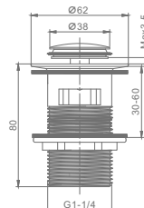
Артикул : R600.05 Донный клапан для раковины • Цвет - хром
