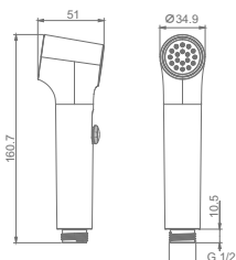
Артикул: R460.05.06 Гигиеническая лейка с клавишей регулировки воды • Цвет - черный
