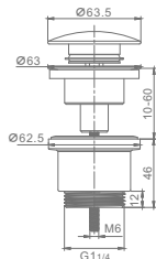
Артикул : R600.01.06 Донный клапан для раковины • Цвет - черный
