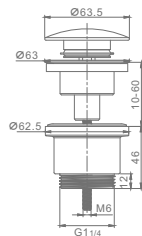
Артикул : R600.01.03 Донный клапан для раковины • Цвет - сатин золотой
