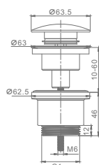
Артикул : R600.01.05 Донный клапан для раковины • Цвет - сатин
