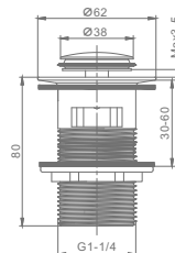
Артикул : R600.05.06 Донный клапан для раковины • Цвет - черный
