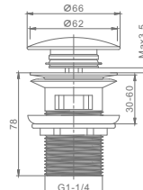
Артикул : R600.03 Донный клапан для раковины • Цвет - хром
