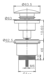
Артикул : R600.01.04 Донный клапан для раковины • Цвет - бронза
