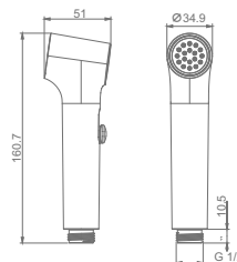
Артикул: R460.05.03 Гигиеническая лейка с клавишей регулировки воды • Цвет - сатин золотой
