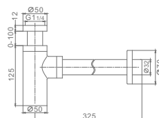
Артикул : R600.20.23 Сифон для раковины • Цвет - золото
