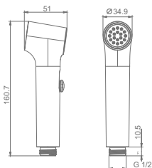
Артикул: R460.05 Гигиеническая лейка с клавишей регулировки воды • Цвет - хром
